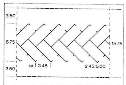
Fig. 9 Fischgrät En arêtes 58 Autos/100 m; 27,2 m 2 /Auto
