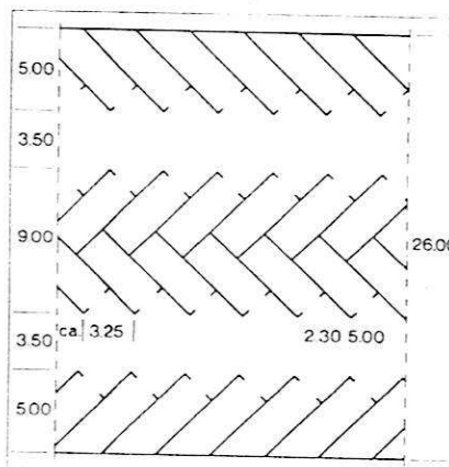
Fig. 8 Fischgrät En arêtes 124 Autos/100 m; 21,1 m 2 /Auto
