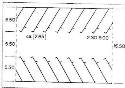
Fig. 7 45° einseitig 45° sur un côté 31 Autos/100 m; 27,6 m 2 /Auto
