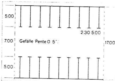
Fig. 4 60° beidseitig 60° sur deux côtés 74 Autos/100 m; 21,9 m 2 /Auto
