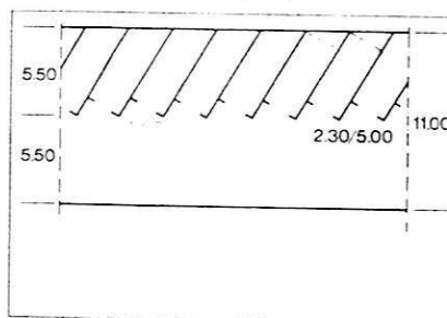
Fig. 8 Fischgrät En arêtes 124 Autos/100 m; 21,1 m 2 /Auto
